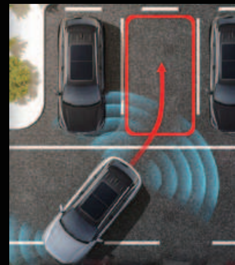
Asistente de estacionamiento automático (APA), con 12 sensores ultrasónicos y 4 cámaras.
